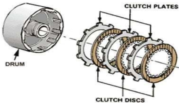
Fig: CLUTCH PACKS
